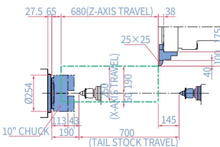
OD HOLDER
