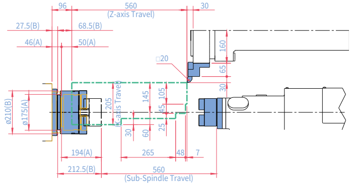
DOUBLE OD HOLDER
