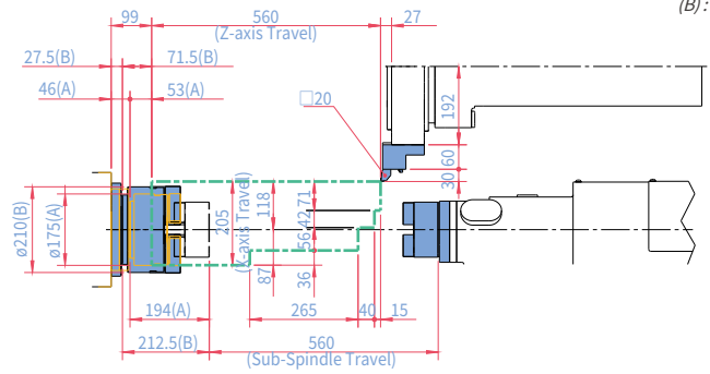
OD HOLDER
